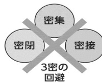
3密の回避
